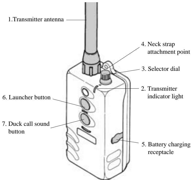
dogtrà RRD transmitter
